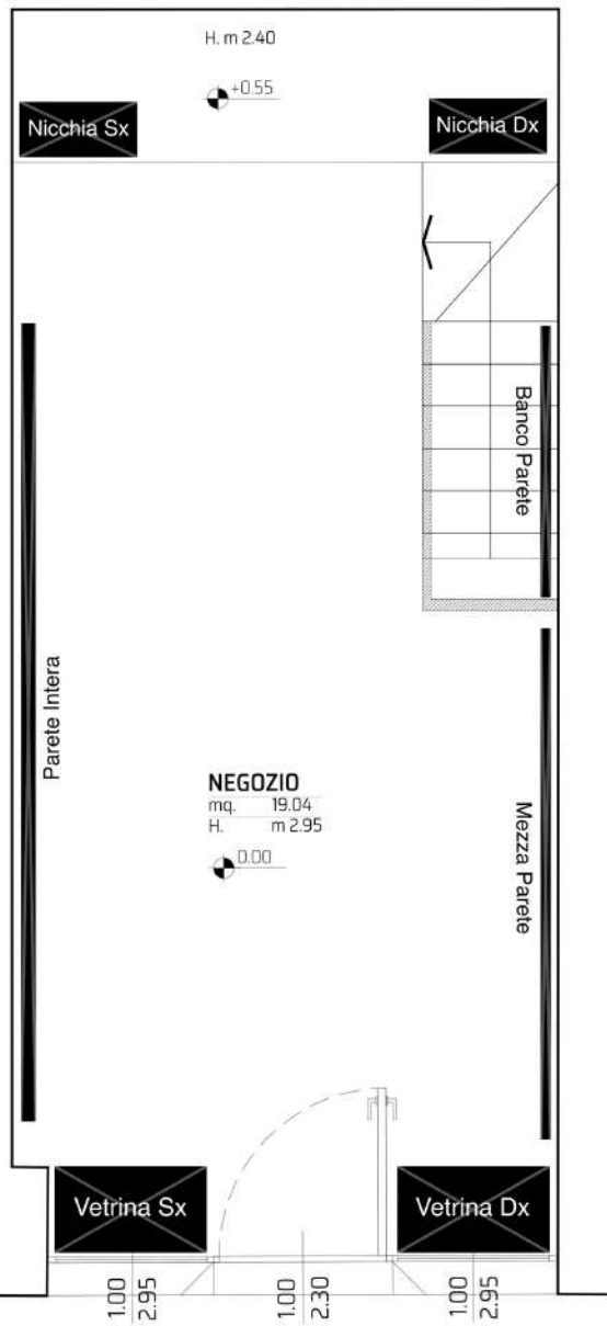
PLANIMETRIA PIANO TERRENO
